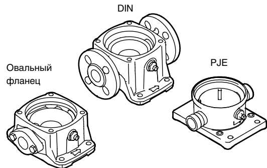
Рис. 33. Трубные соединения насоса.
