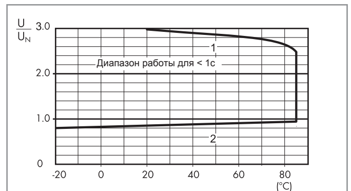
R 67 - Отношение рабочего диапазона к температуре окр. среды, 67.хх-4300/4500 в режиме энергосбережения (-40...+85)°C
