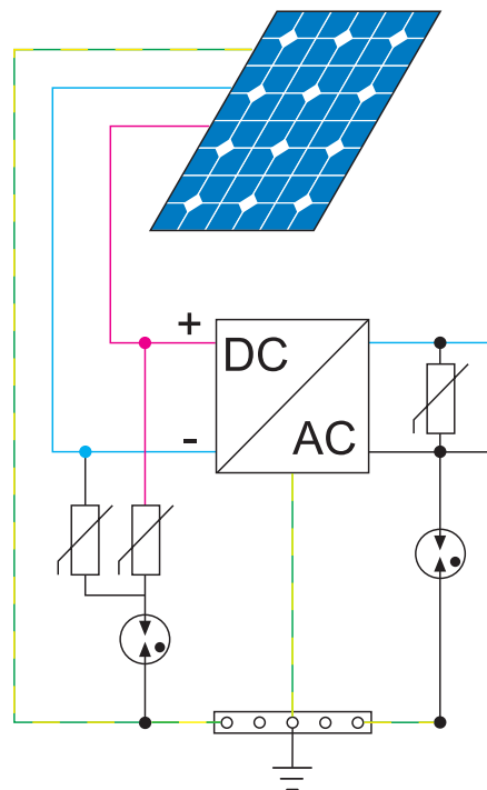
Рис 10: пример фотогальванической системы для здания не оборудованного системой защиты от молнии; защита со стороны DC при помощи УЗИП с U_{oc stc} = 420 В, и защита со стороны AC устройством 7P.22, характерным для систем TT.
