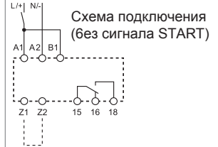
Схема подключения (без сигнала START)
