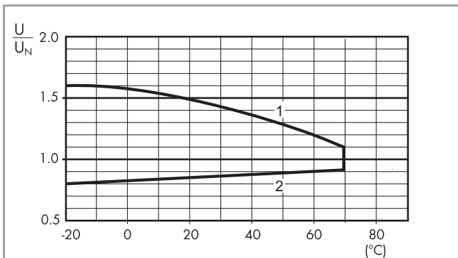
R 67 - Отношение рабочего диапазона к температуре окр. среды, 67.хх-4300 при стандартном питании катушки (постоянно) (-40...+70)°C
