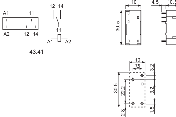
Вид со стороны выводов
