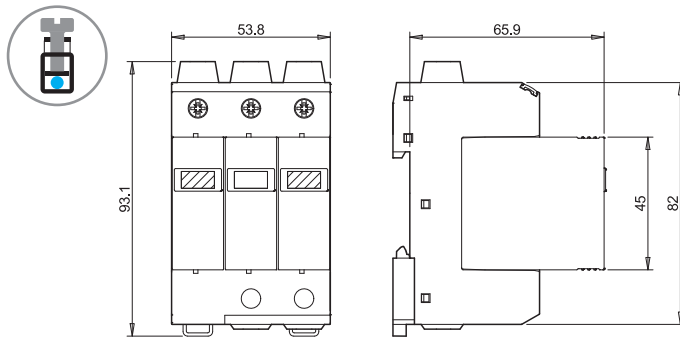
Тип 7P.26.9.000.1015 Винтовые клеммы
