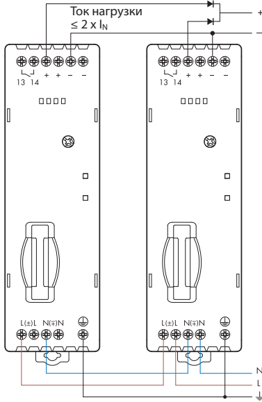
Параллельное подключение
