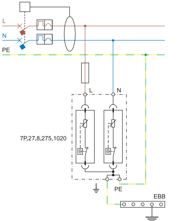
TN-S ОДНОФАЗНАЯ СИСТЕМА - УСТАНОВКА УЗИП ПОСЛЕ УЗО
