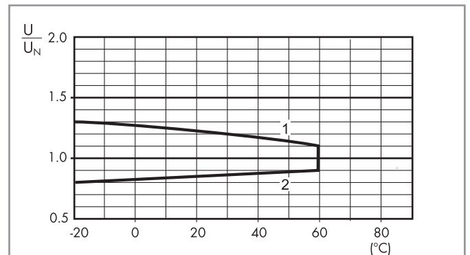
R 67 - Отношение рабочего диапазона к температуре окр. среды, 67.хх-4500 при стандартном питании катушки (постоянно) (-40...+60)°C
