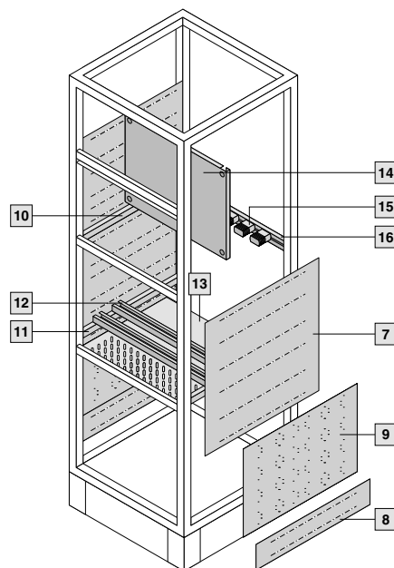
Оборудование секции
