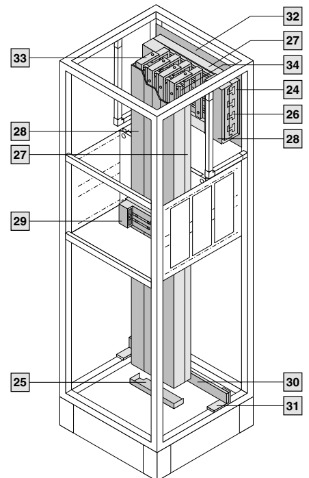
Шинные системы
