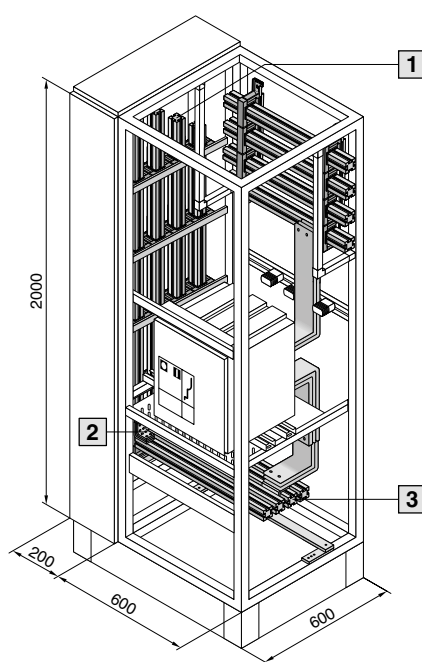
Шинные системы
