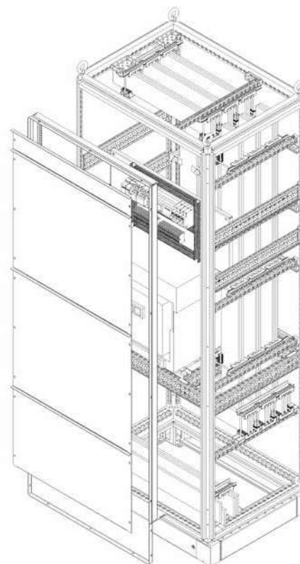
Пластронная система
