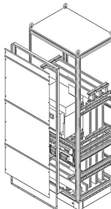
Пластиковая система
