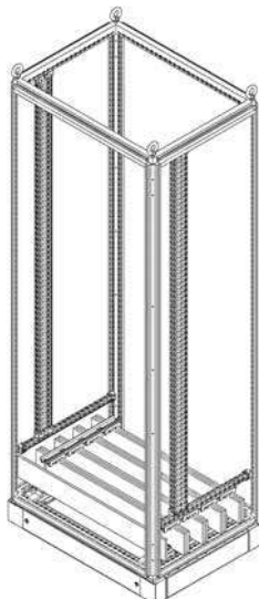
Шинные сборки
