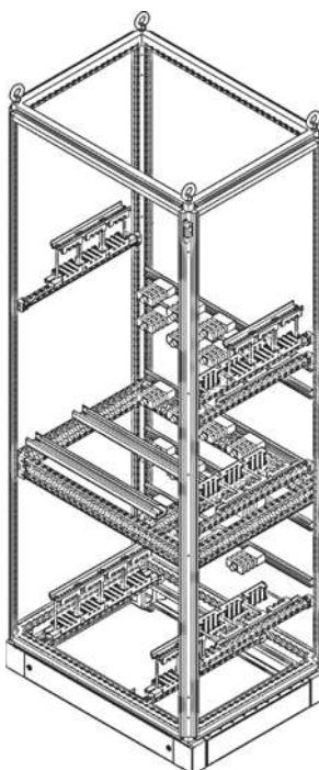
Шинодержатели
