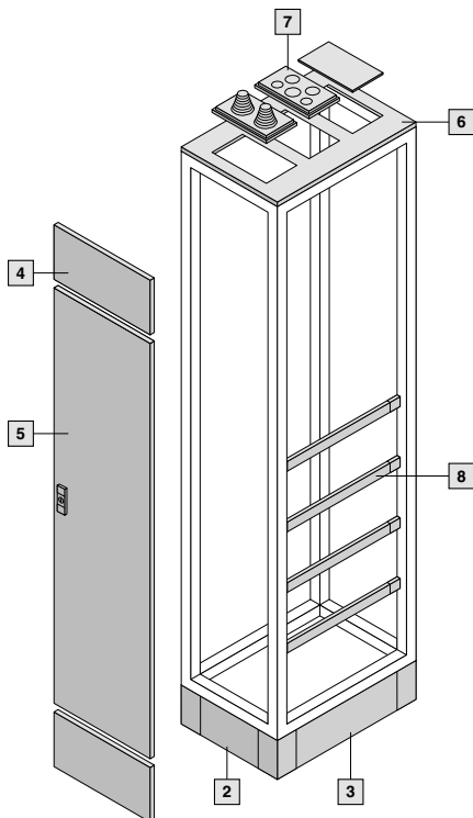
Комплектующие шкафа
