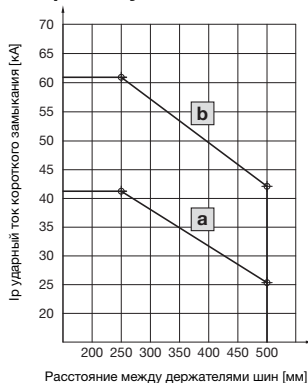
Диаграмма устойчивости к короткому замыканию
