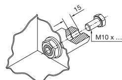
Крепление снаружи
