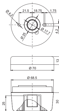
Элемент подключения для настенного/напольного монтажа 2368.010
