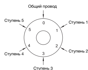
Схема подключения
