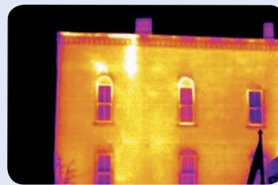
Эксфильтрация воздуха
