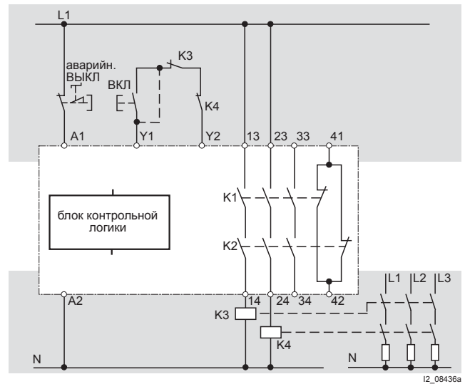
Присоединение внешних контактов
