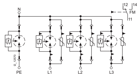
4-полюсные 5SD7 444-1
