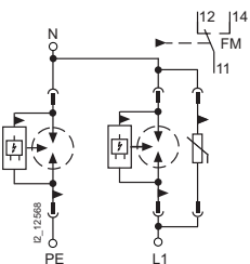
2-полюсные 5SD7 442-1
