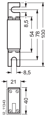
3NE1 2...-0, 3NE1 2...-2
