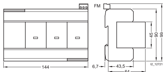
3-полюсные 5SD7 413-1
