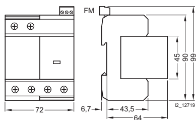
3-полюсные 5SD7 413-1
