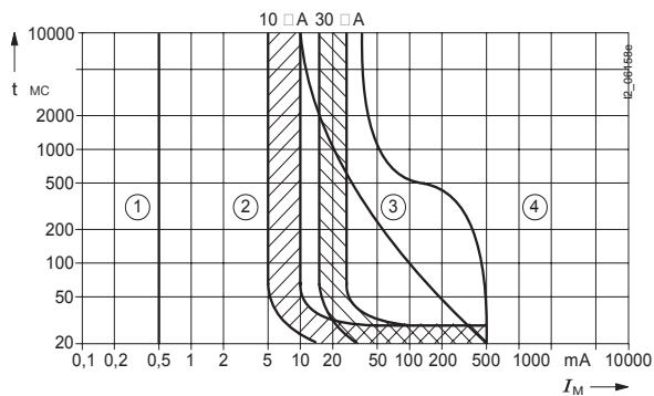
Диапазоны силы тока по МЭК 60 479
