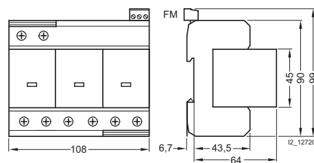
4-полюсные 5SD7 414-1
