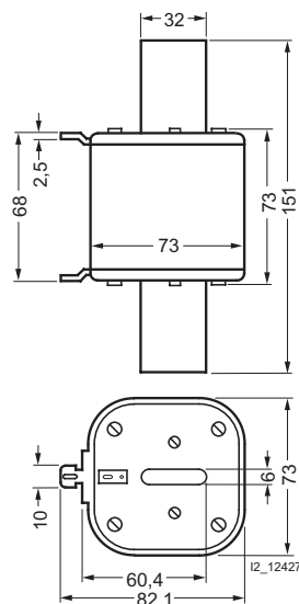
3NE1 4...-2
