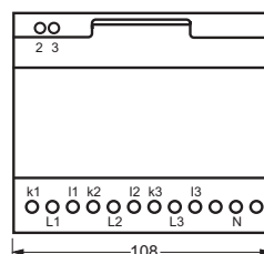
7КТ1 301
