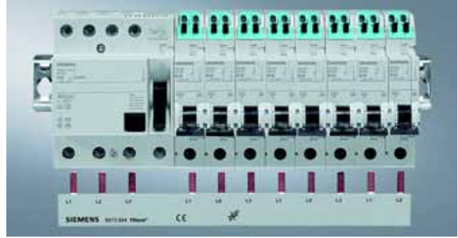
Подключение автоматических выключателей к 4-полюсному УЗО (N-зажим слева) распливаемой 3-полюсной сборной шиной из программы 5ST3 7..
