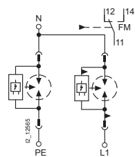
2-полюсные 5SD7 412-1
