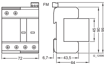
2-полюсные 5SD7 442-1
