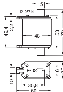
3NE1 02...-0, 3NE1 02...-2, 3NE8 0...-1
