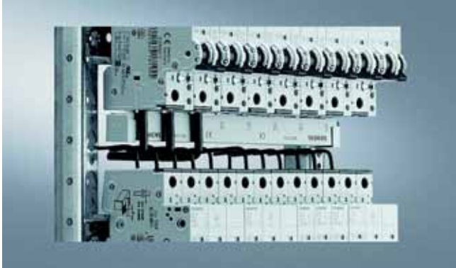
Оптимальное пространство для монтажа также и при малых расстояниях между монтажными рейками
