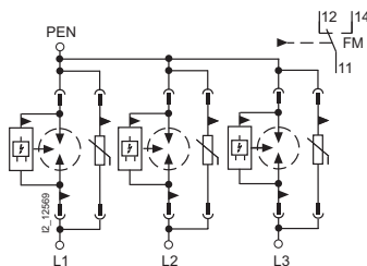
3-полюсные 5SD7 443-1
