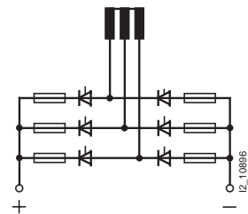
шестипульсная мостовая схема B6 с предохранителями в ветвях
