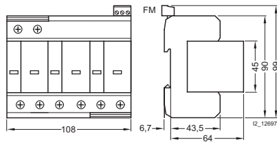
3-полюсные 5SD7 443-1
