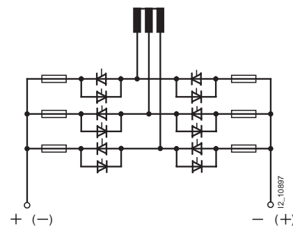
шестипульсная мостовая схема B6 с предохранителями в ответвлениях (реверсивная схема)
