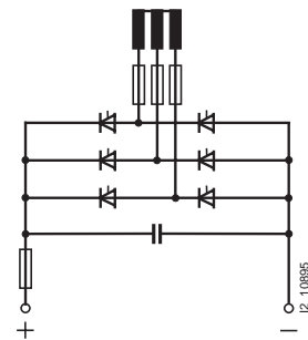
шестипульсная мостовая схема B6 с фазными предохранителями и предохранителем постоянного тока (схема для преобразователя частоты переменного тока)
