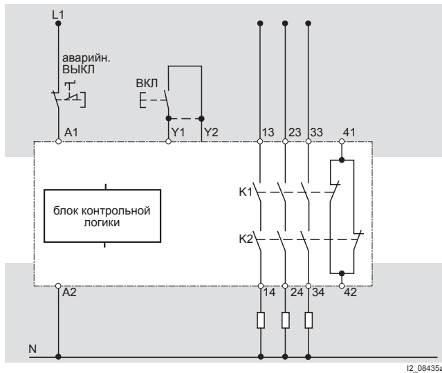
Прямое подключение 230 В/400 В до 5 А
