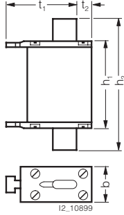
типоразмер 4 (конструктивное исполнение МЭК)
