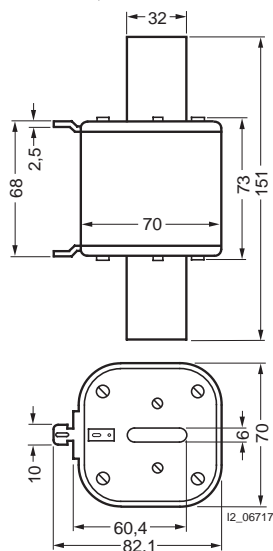
3NE1 43...-0, 3NE1 43...-1
