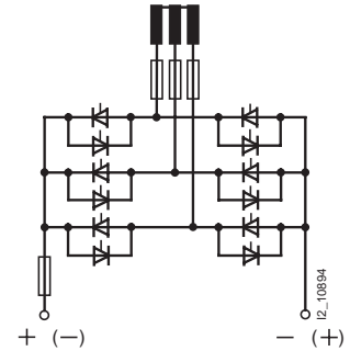
шестипульсная мостовая схема B6 с фазными предохранителями и предохранителем постоянного тока (реверсивная схема)
