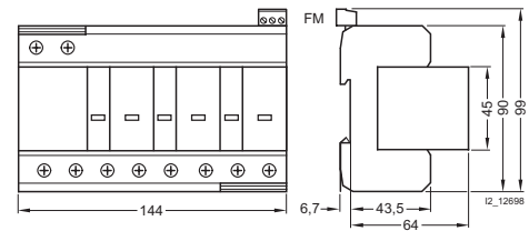
4-полюсные 5SD7 444-1
