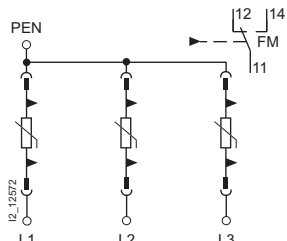
5SD7 423-0 без телесигнализации (FM)
