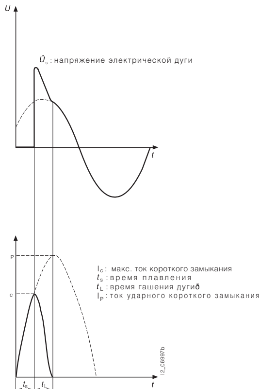
Осциллограмма отключения тока короткого замыкания плавкой вставкой предохранителя
