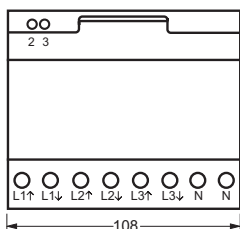
7КТ1 302
