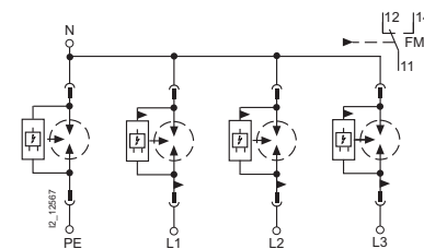
4-полюсные 5SD7 414-1
