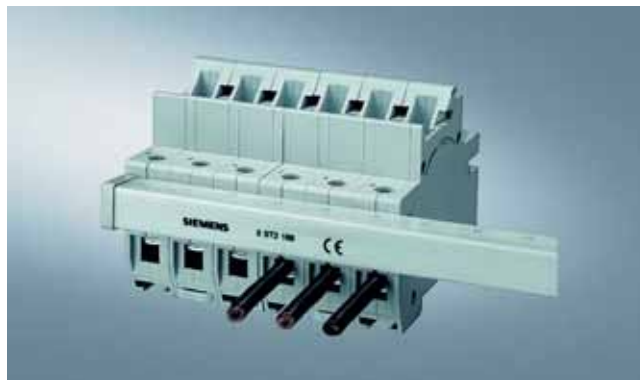
предохранители-выключатели нагрузки 3-полюсные 5SG7 630 сборная шина 5ST2 188 или 5ST2 192 торцевые крышки 5 ST2 177
