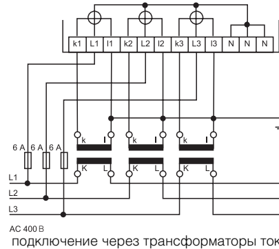
AC 230 / 400 В подключение через трансформаторы тока, 4-проводная схема
