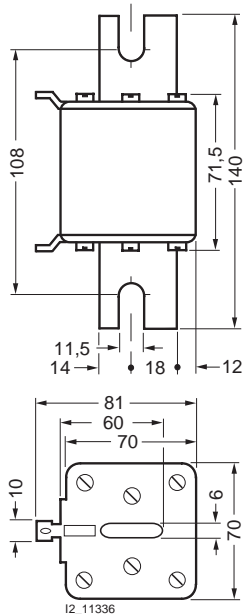
3NC2 4...-3, 3NC8 4...
