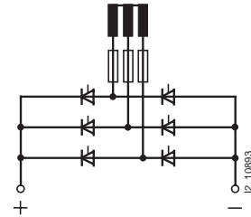
шестипульсная мостовая схема B6 с фазными предохранителями
