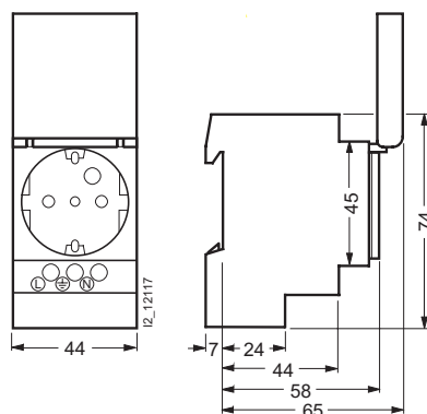
5TE6 802
