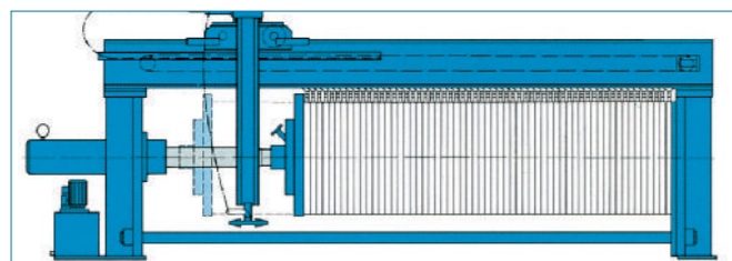
Гидравлическая система закрытия с помощью сжимающего цилиндра для плит размером до 2000 x 2000 мм и давлений фильтрации до 60 бар.
