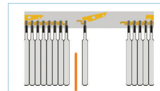
Бесконечная цепь со сцепленными плитами для быстрого открытия фильтрпресса
