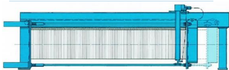
Гидравлическое закрытие с помощью притягивающего цилиндра для плит размером до 2450 x 2450 мм и давлений фильтрации до 50 бар.
