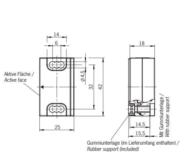
Betätiger/Actuator
