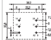
62.22 - 0300 Вид сбоку
