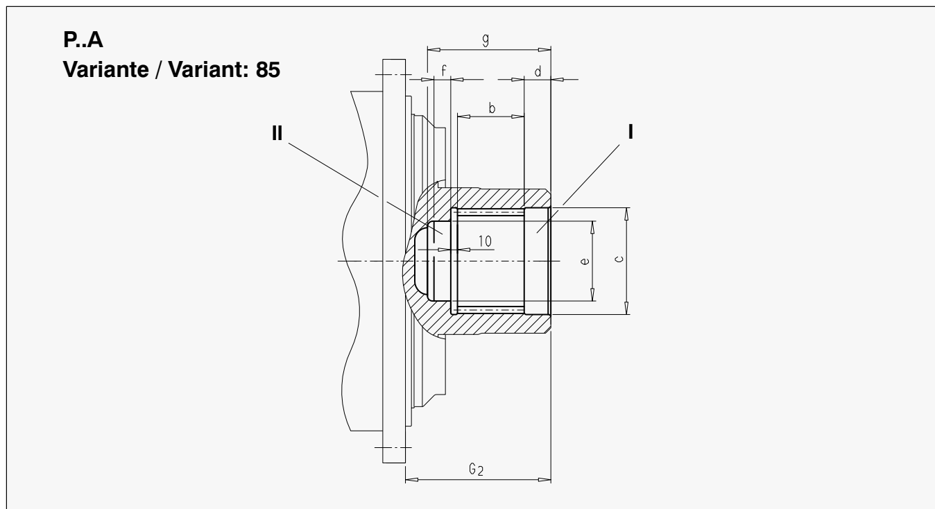
Maße und Gewichte / Dimensions and weights / Dimensions et poids
