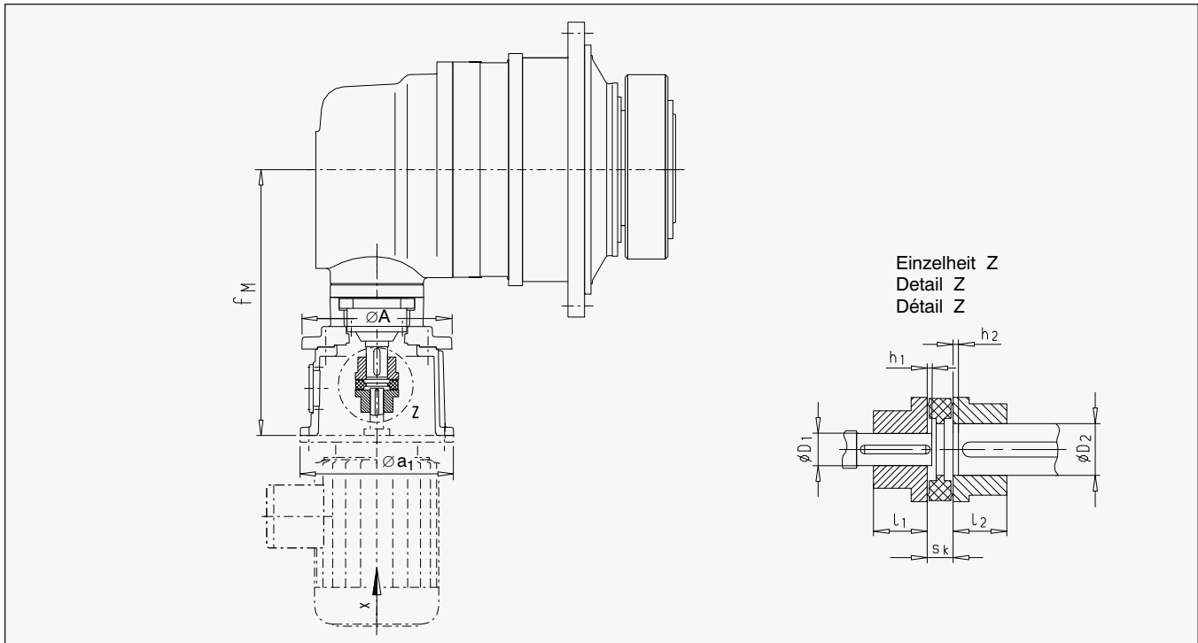
Maße / Dimensions / Dimensions
