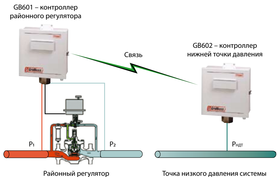
Компоненты GridBoss
