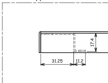
Деталь X
