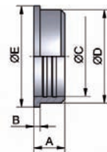
SMS-Nutmutter
