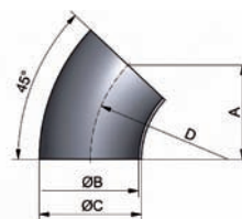
welding bend DIN 11852-BS 45° CC
