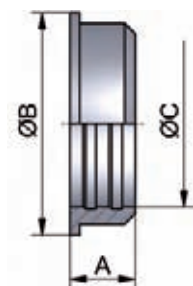
DS-Nutmutter
