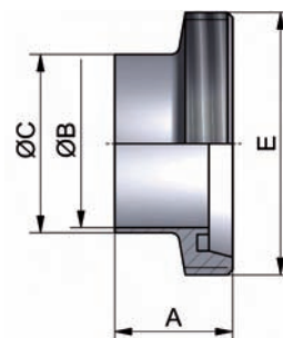
Kegelstutzen Zoll
