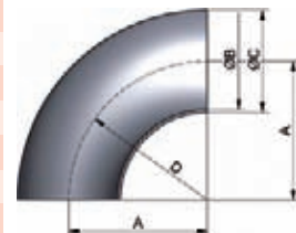
welding bend DIN 11852-BS 90° CC
