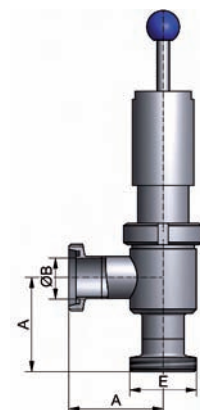
Überström-Eckventil GG-federbelastet angle-body relief valve male/male spring loaded
