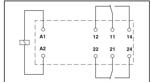
Реле с 2 переключающими контактами и ручным управлением, макс. 2 x 8 А
