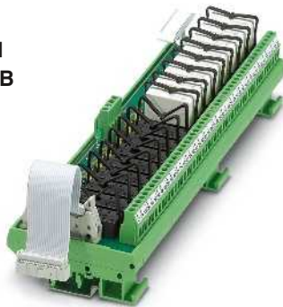
Модуль вывода и расширения с 16 миниатюрными реле, 1 переключающий контакт
