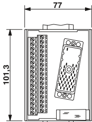
Чертеж UMK-EC56/32-XOR
