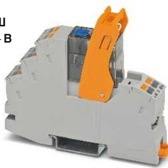
Релейный модуль с 2 переключающими контактами с зажимом push-in и ручным управлением
