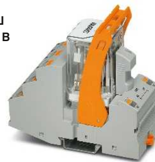
Мощный релейный модуль с 2 переключающими контактами с зажимом push-in
