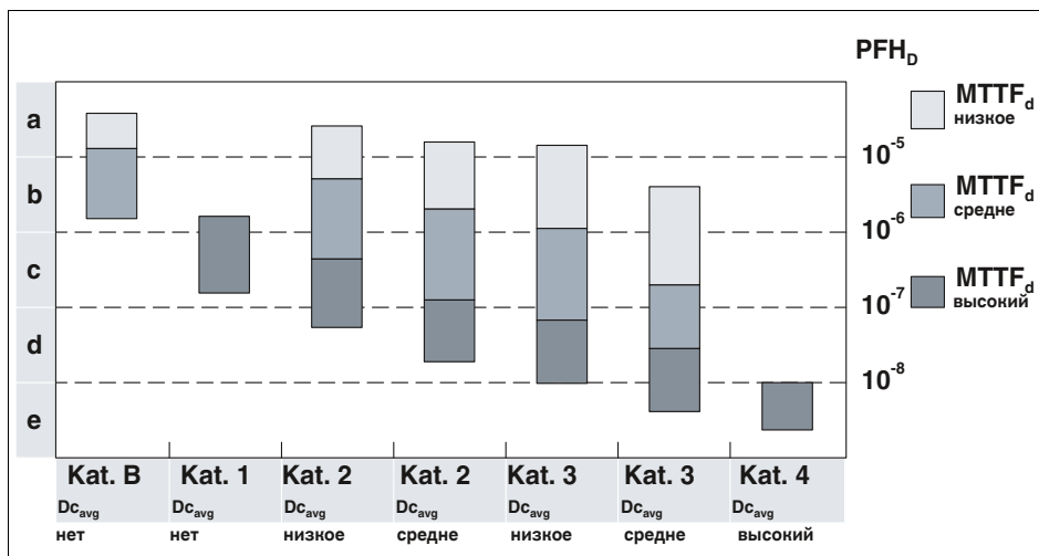
Рис. 5: Связь PL, категории, DC и MTTFd (согласно EN 13849-1)
