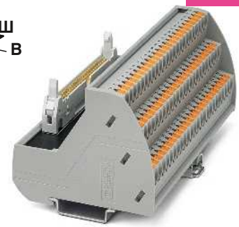
50-конт. штыревая планка IDC/FLK с потенциалами P1 и P2
