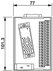
Чертеж UMK-EC56/32-XOL
