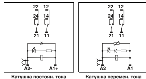
Катушка постоянн. тока
