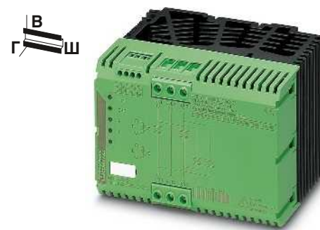
для реверсирования 3-фазных двигателей переменного тока до 575 В перем. тока/3 x 37 А
