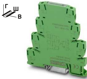
Модуль полупроводникового реле, выход пост. тона макс. 500 мА, с электронным переключающим контактом
