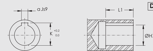
Keyway / Clavetage : NFE 22175
