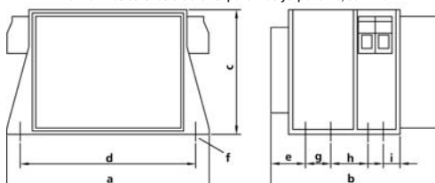
Компактное сетевое стабилизированное устройство, 36 – 120 Вт
