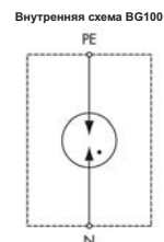
Внутренняя схема BG100 газовый защитный разрядник нейтрали/заземления
