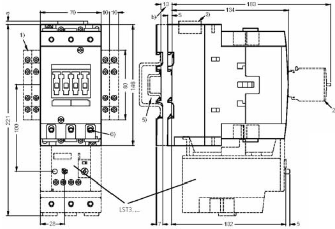
LSD3.... размер S3
