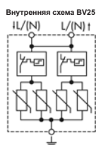
Внутренняя схема BV25 Внутренняя схема BVR 25-275* варистор
