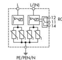
Внутренняя схема VVR
